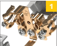
1 токоведущая часть выполнена из оловянно- фосфорной бронзы
